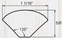
54WSQN END CAP
